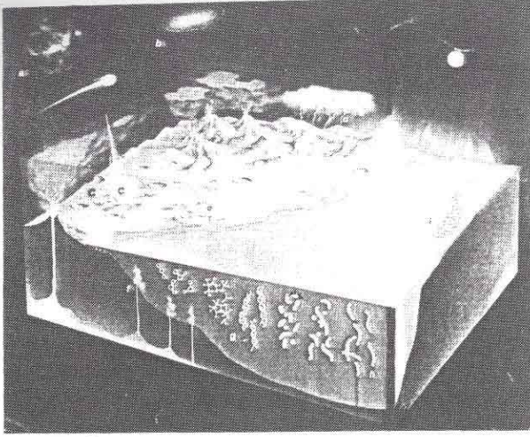
Şekil 2. Güneş sistemi bundan 4.5 milyar yıl kadar önce bir gaz ve toz bulutunun yoğunlaşması ile başladı (a,b). Organik maddeler göktaşları ile taşınarak (c), atmosferde (d), deniz kenarındaki med-çezir göllerinde (e) veya denizlerin derinliklerindeki ısı kaynaklarında (f) meydana geldi. Bu kimyasal maddeler birleşerek proteinler ve nükleik asitler gibi daha karmaşık molekülleri oluşturdu (g). 3.5 milyar yıl kadar önce fotosentez yapabilen mikroplar meydana geldiler (h). Bu ilkel organizmalar sığ denizlerin kıyılarında stramatolitler tepelikleri oluşturdu (i).
